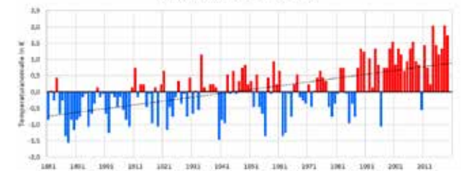
Abweichungen Temperatur für NRW in Kelvin gegenüber Mittelwert Klimanormalperiode 1961 - 1990
